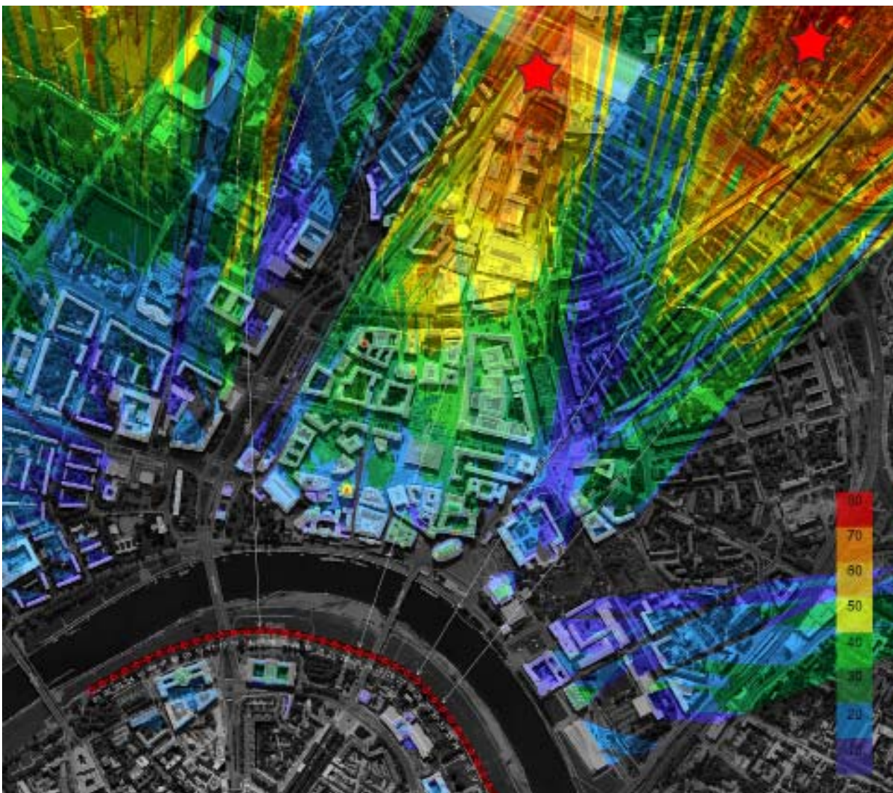
Il. 6. Wynik analizy VPS uwzględniającej pełną ochronę panoram nadrzecznych Drezna. W polu mapy maksymalna wysokość zabudowy wynosi 80m. Każdy wyższy budynek będzie widoczny w panoramach z nad rzeki (il. autorów)
